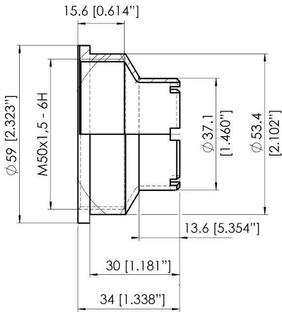
PN: AVE-BMBP-150 - Ball Vent Bottom Part 1 ½"
