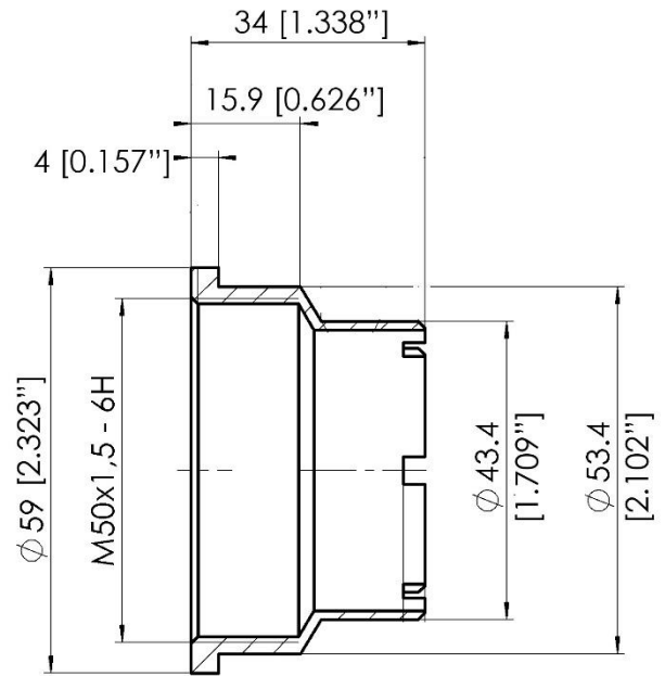
PN: AVE-BMBP-175 - Ball Vent Bottom Part 1 ¾"
