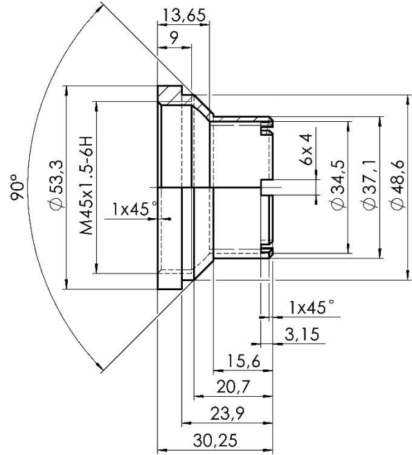
PN: AVE-BVBP-150 - Ball Vent Bottom Part 1 1/2"
